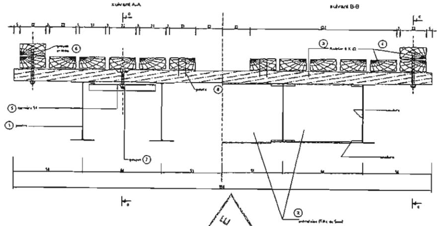
Coupe transversale
