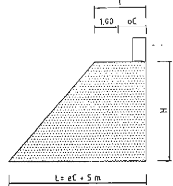
COUPE B-B
