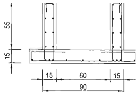
CANIVEAU DOUBLE
