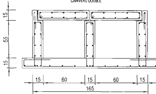
CANIVEAU DOUBLE
