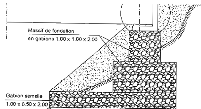
COUPE A-A
