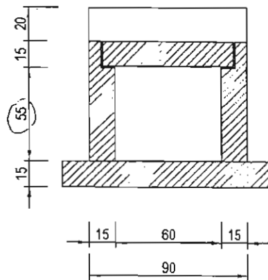
COUPE TRANSVERSALE
