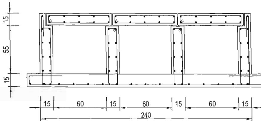
CANIVEAU TRIPLE
