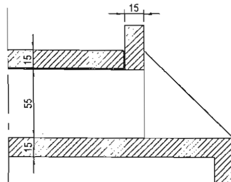
COUPE LONGITUDINALE
